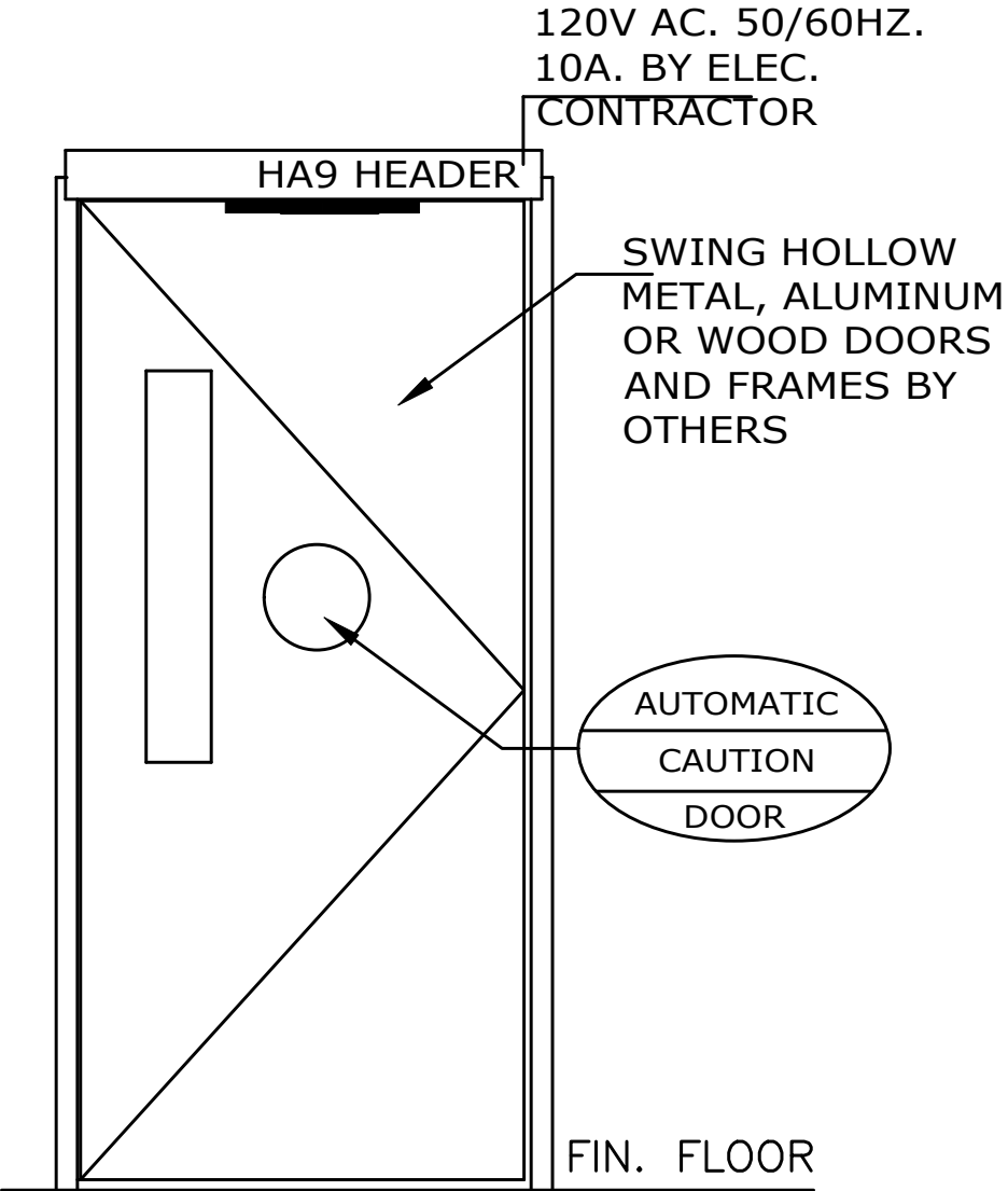
ELEVATION
