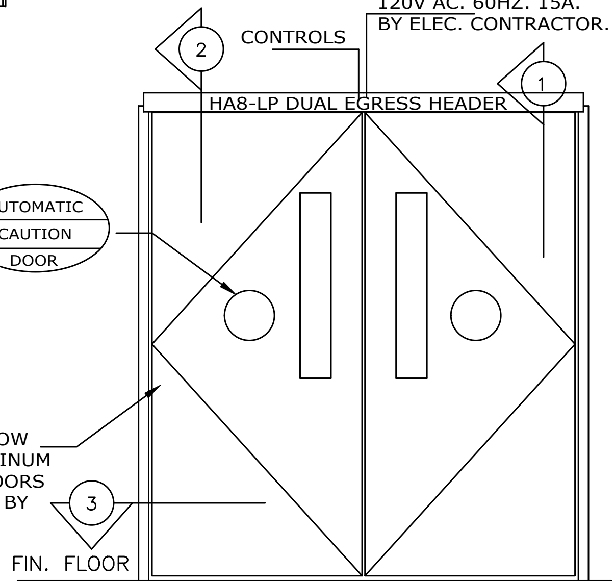
ELEVATION
