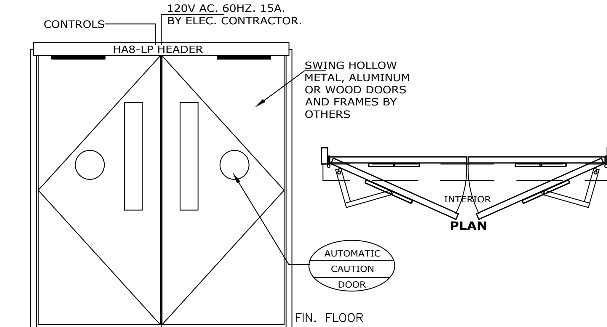
ELEVATION
