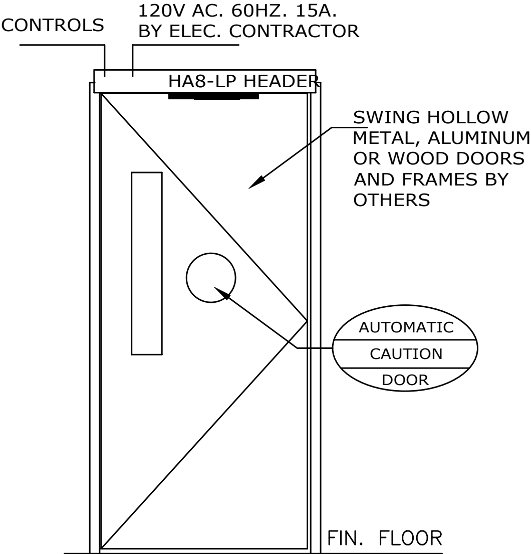
ELEVATION
