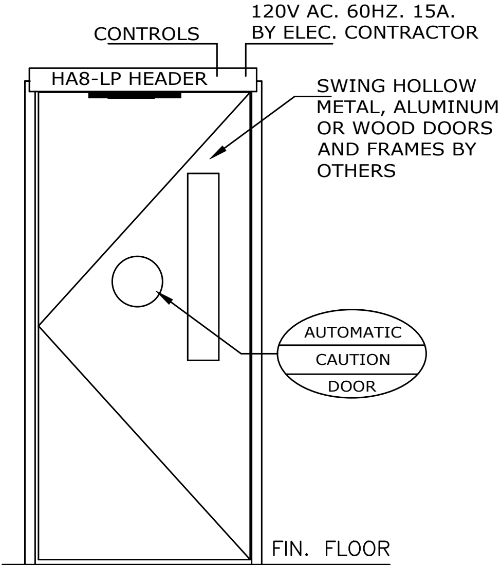
ELEVATION
