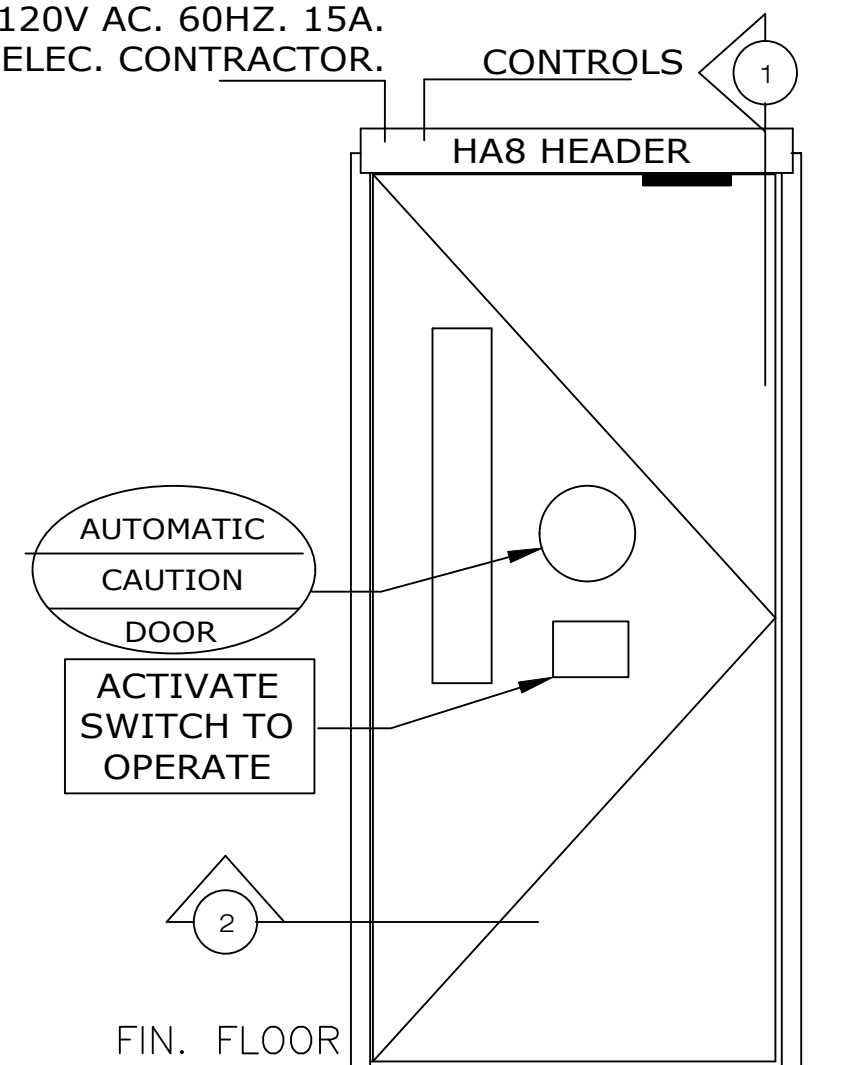
ELEVATION
