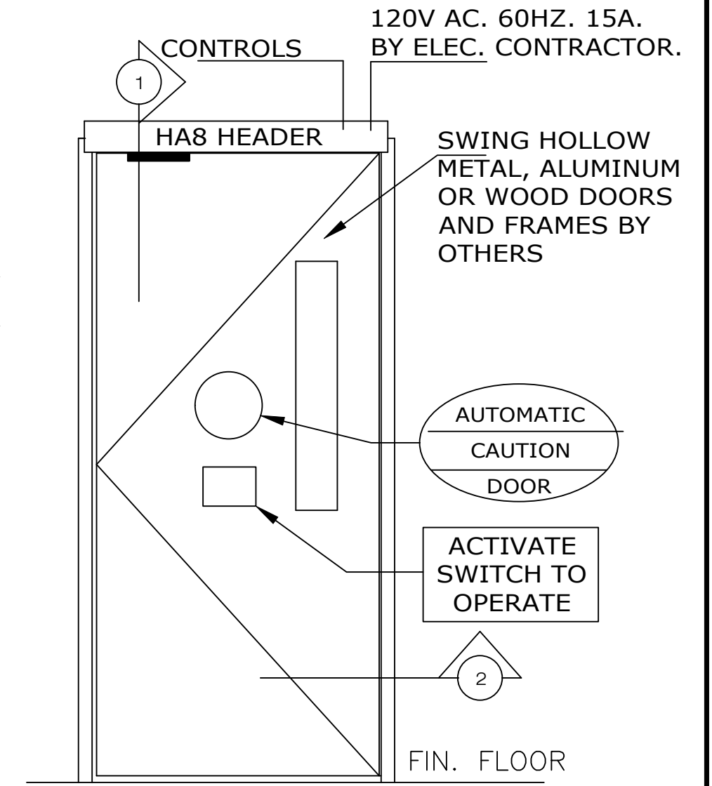
ELEVATION
