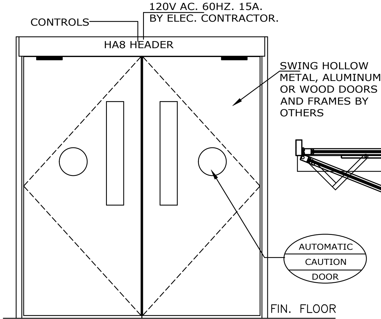
ELEVATION
