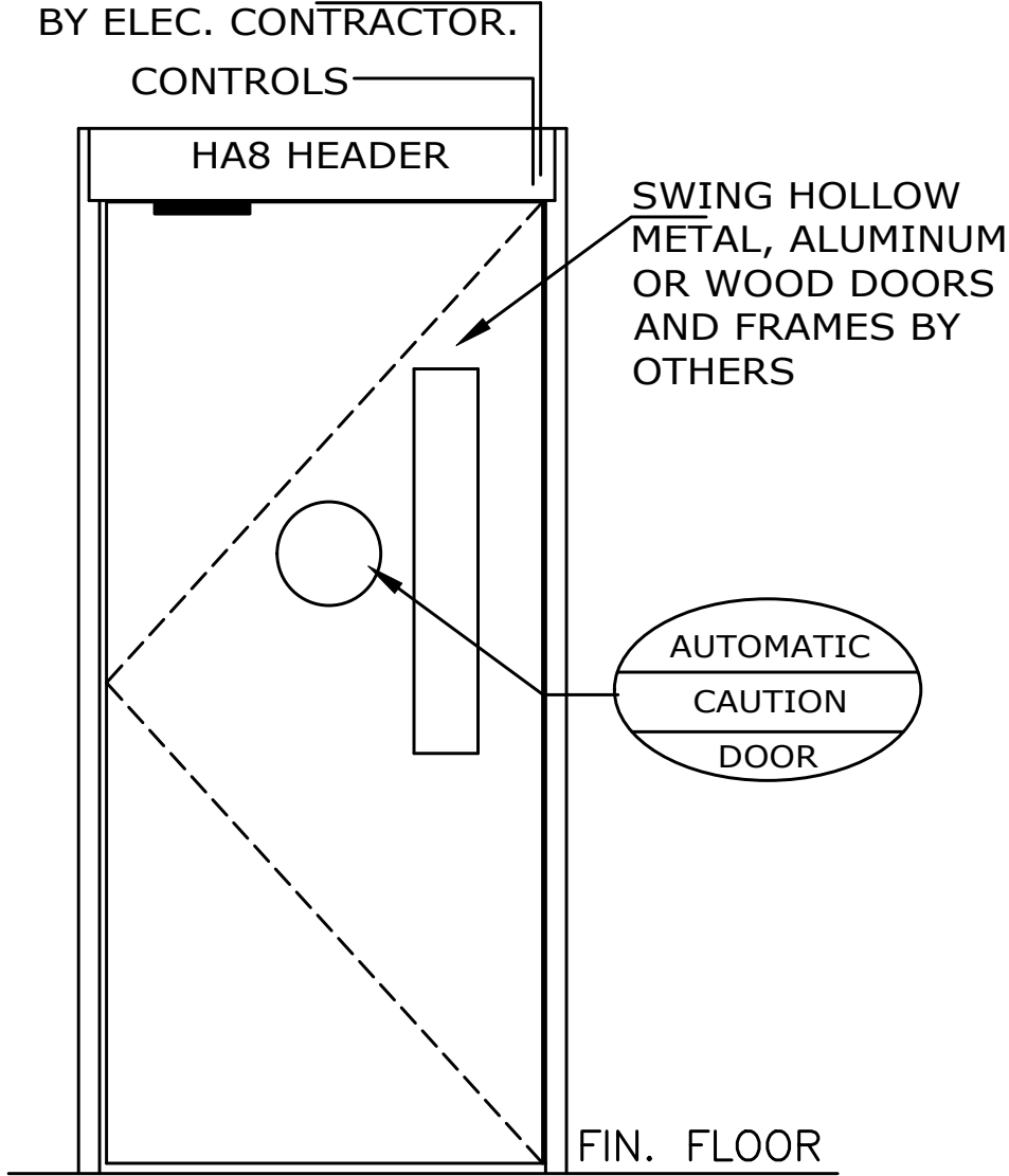
ELEVATION
