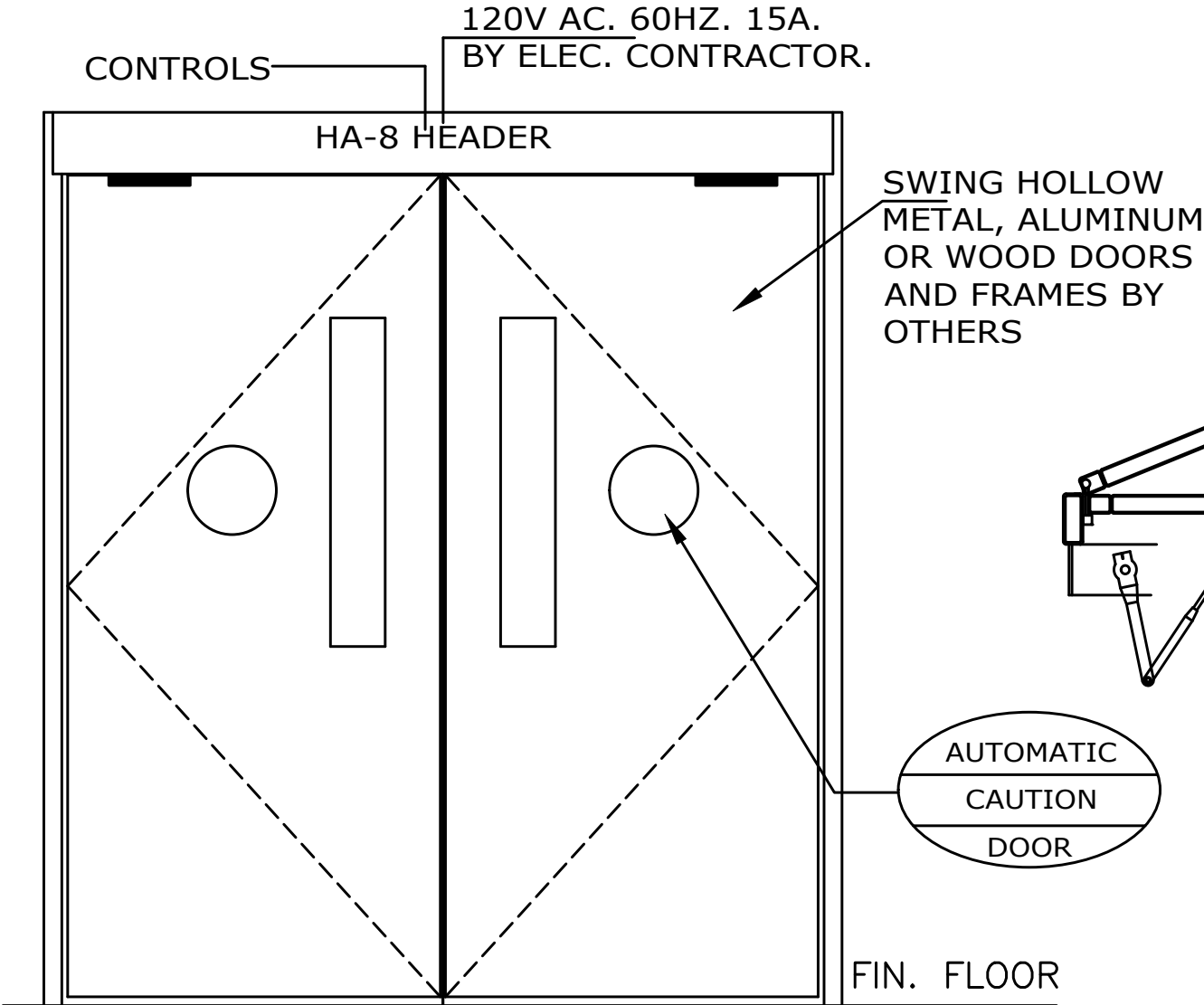
ELEVATION
