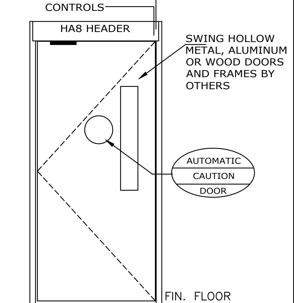
ELEVATION
