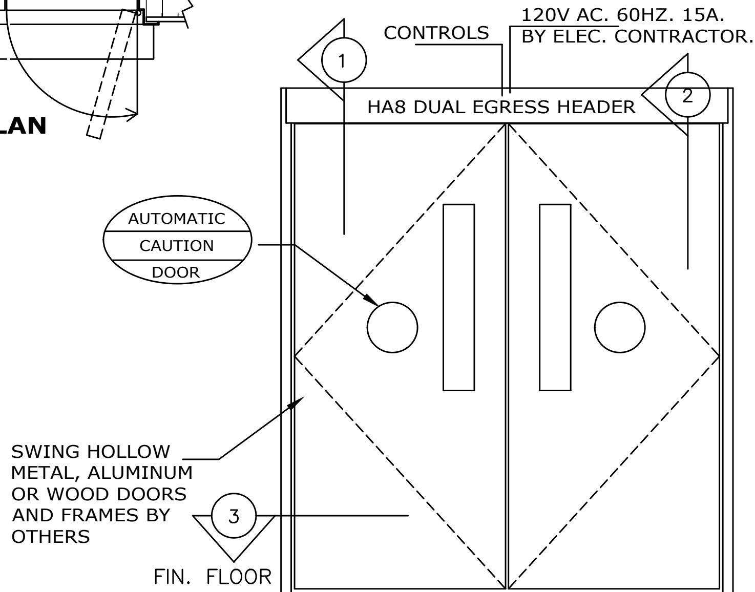
ELEVATION
