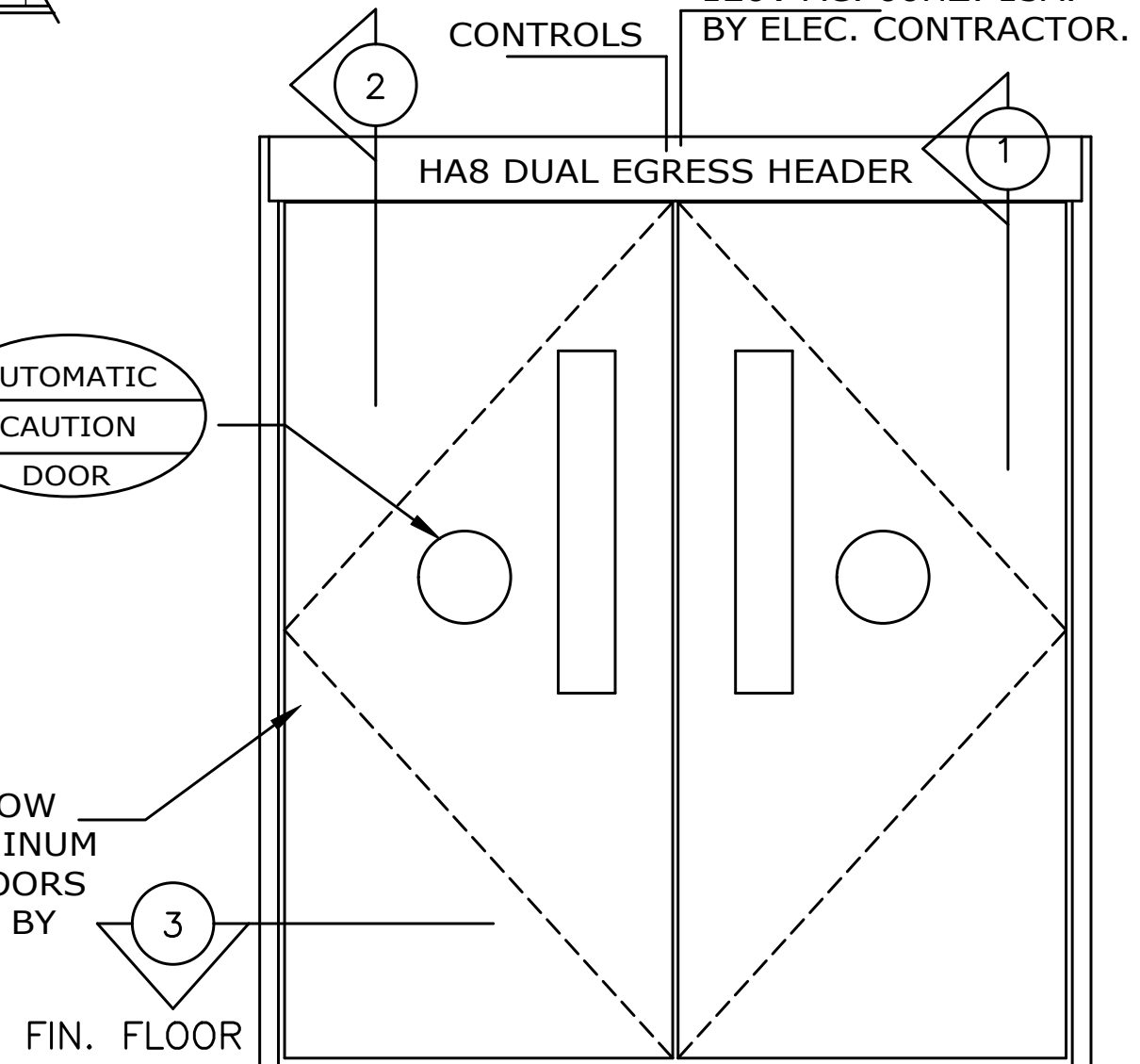
ELEVATION
