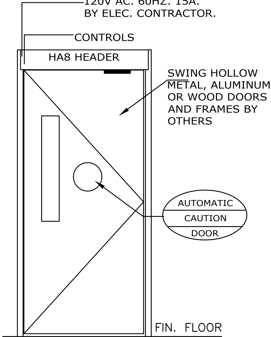
ELEVATION
