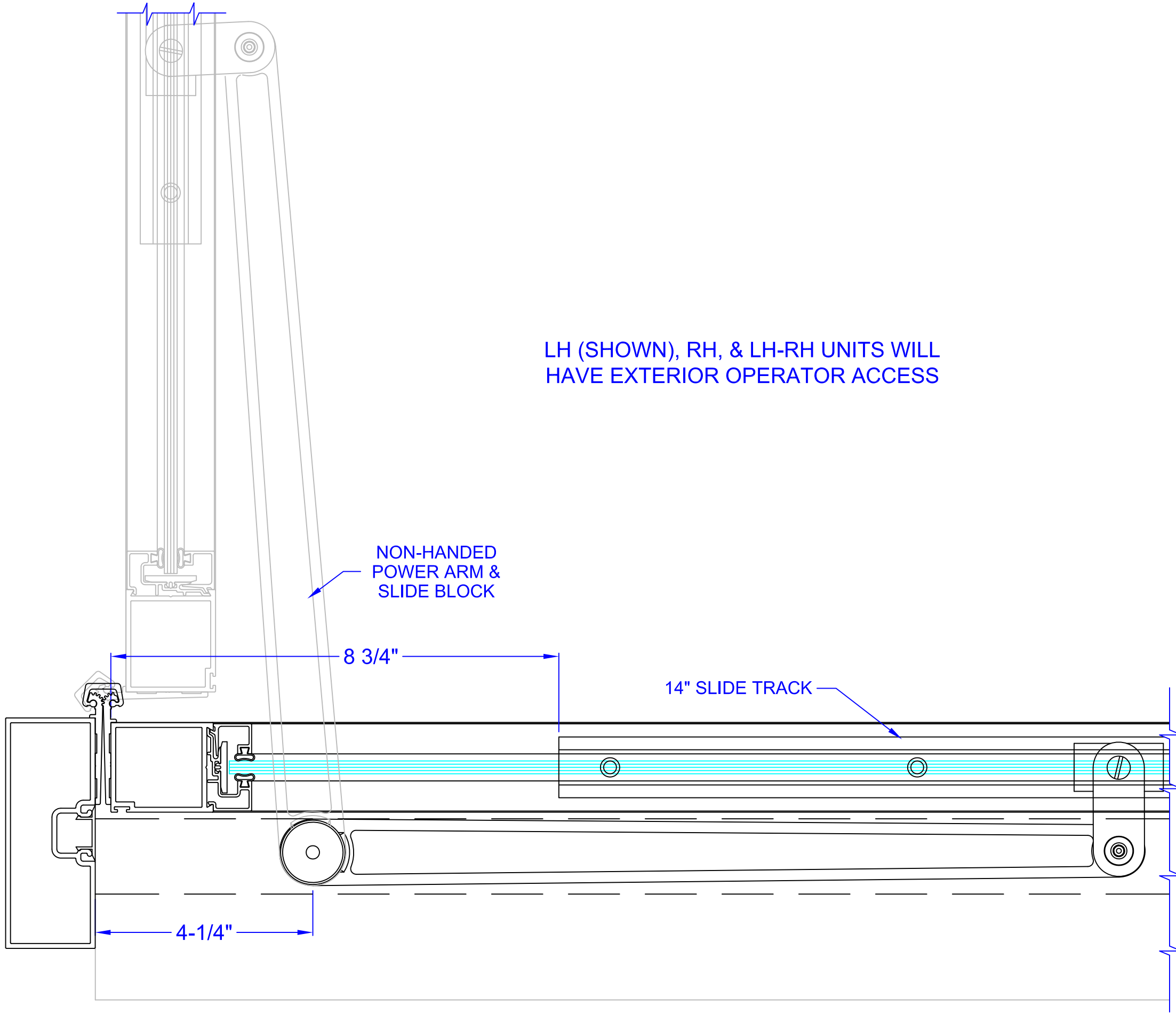
ARM DETAIL SCALE: 1/2 SIZE
